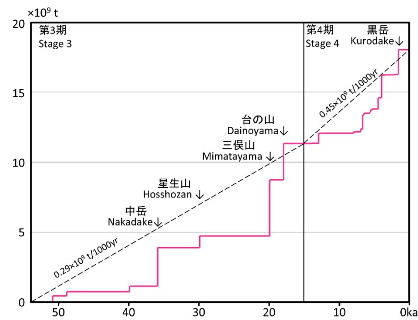
第 3 図 九重火山第 3 期～第 4 期の積算噴出物量段階図. Fig. 3 Cumulative volume diagram of Kuju Volcano from Stage 3 to Stage 4.
