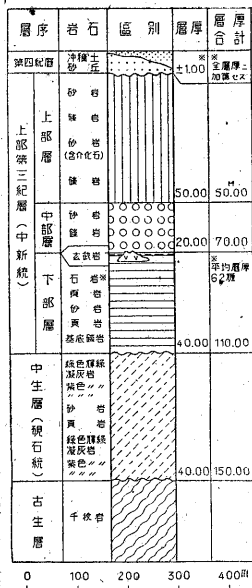
第2図 国分炭礦附近一般地質模式柱状図
