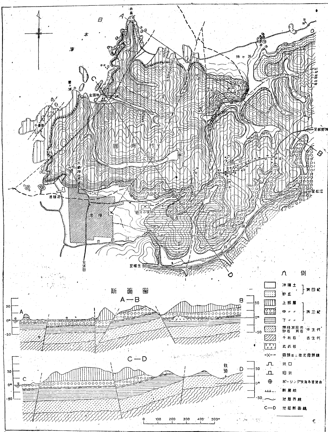
第 1 図 国分炭礦地質図及び断面図
