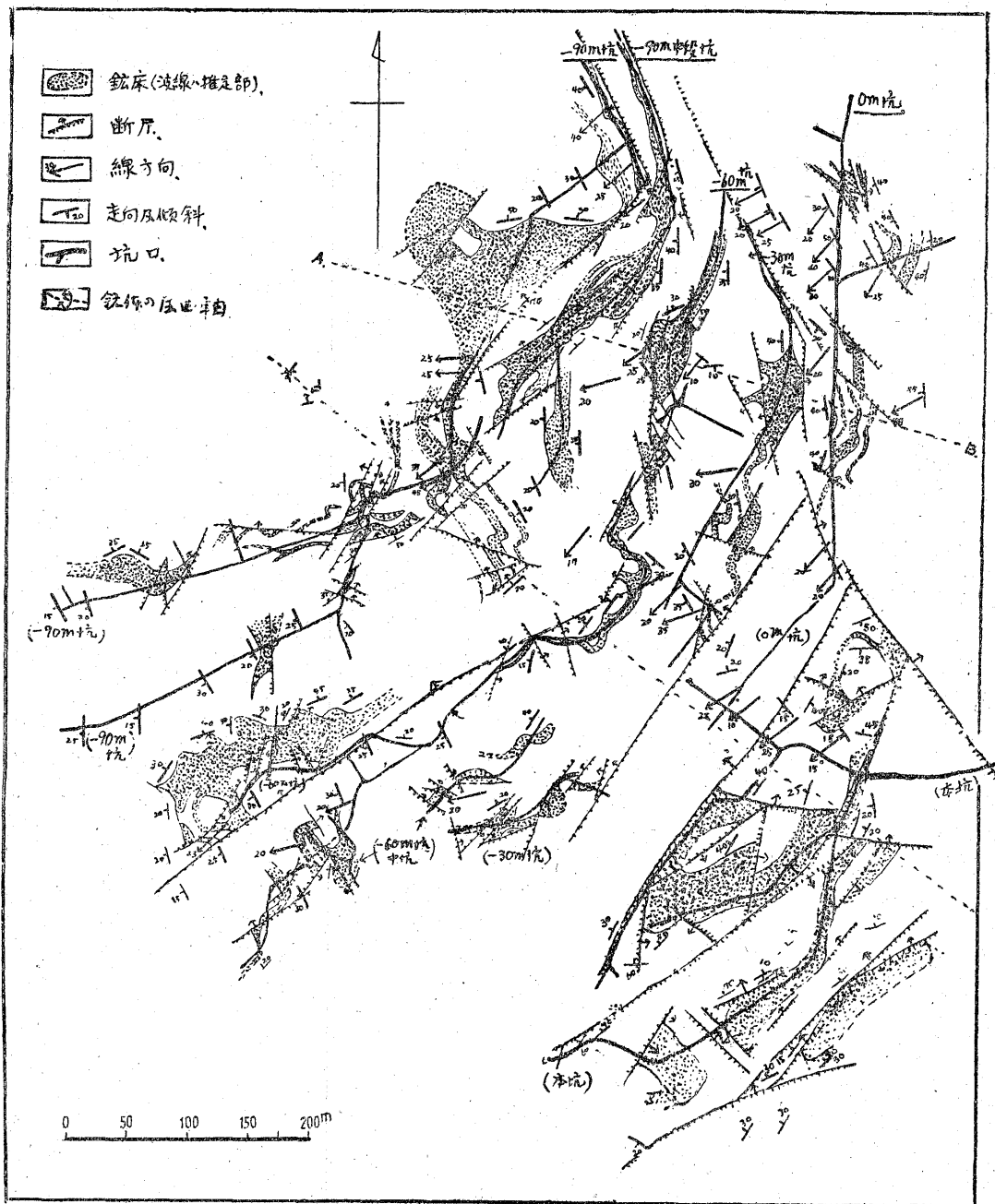
第2図 河山鉾山鉾床図
