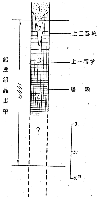
第 4 図 藍内坑種鉍床構造模図 1. 粘土質物 2. 方鉛晶出部 3. 方鉛の多い混合晶出部 4. 混合晶出部
