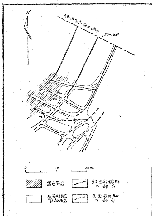
第6図 一番坑中段鑛床見取図
