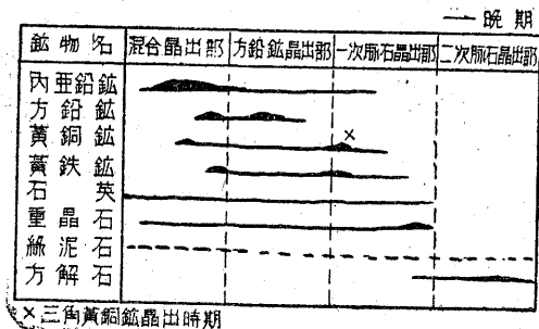
第 3 図 鉍石礦物の晶出順序
