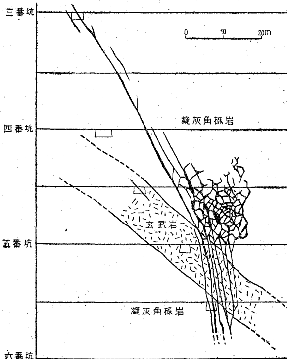
第6図 本坑富鉛床の模式断面図
