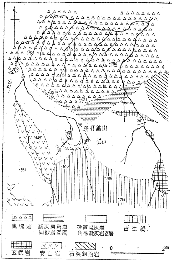
第 2 図 舟打鉍山附近の地質概念図
