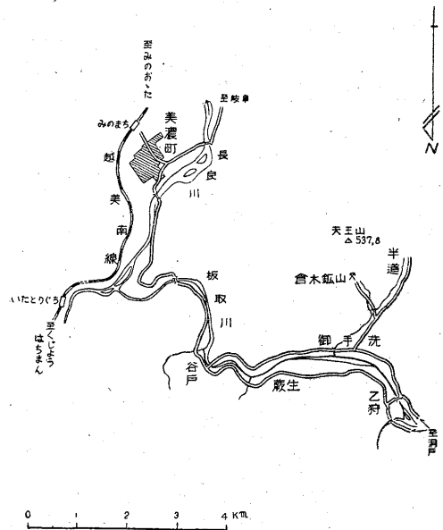
第1図 倉木鉱床位置交通圖
