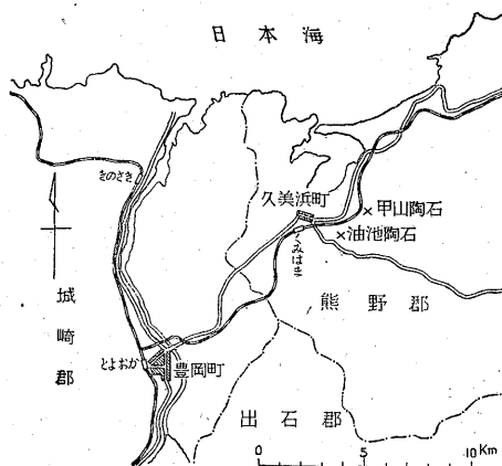
第1図 京都府甲山・油池両陶石鉱床位置図
