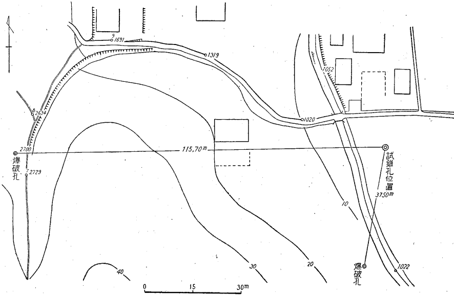
第2図 馬目 Well-Shooting 爆発孔位置図
