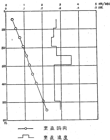
第3図 馬目試錐孔 Well-Shooting 測定結果
