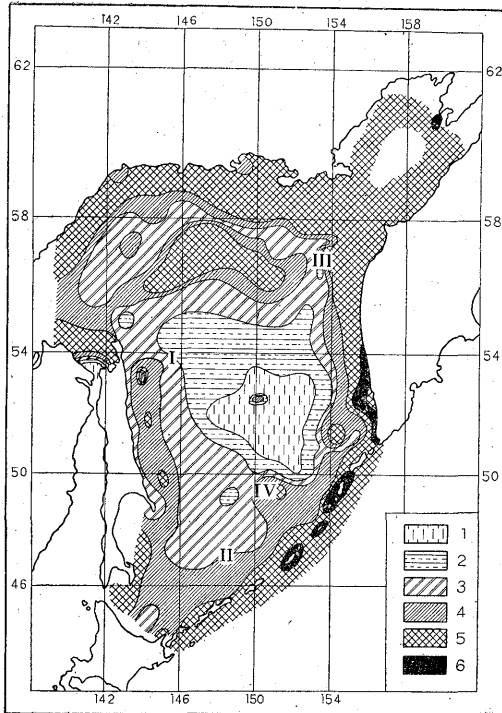
第2図 \text{TiO}_2 の等分布図
