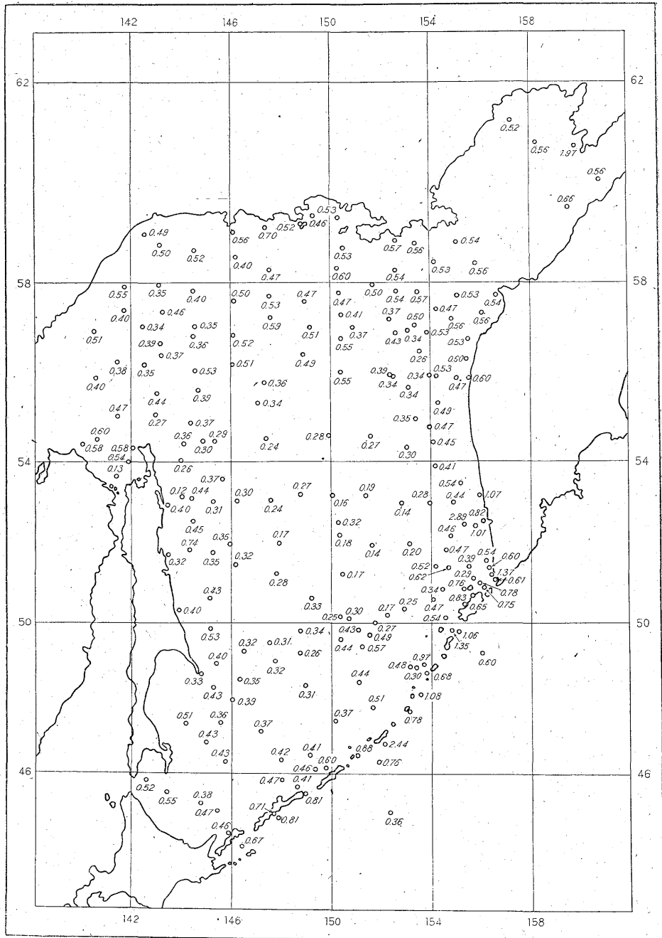
第1図 各試料採取地点の海底堆積中における \text{TiO}_2 の含有量
