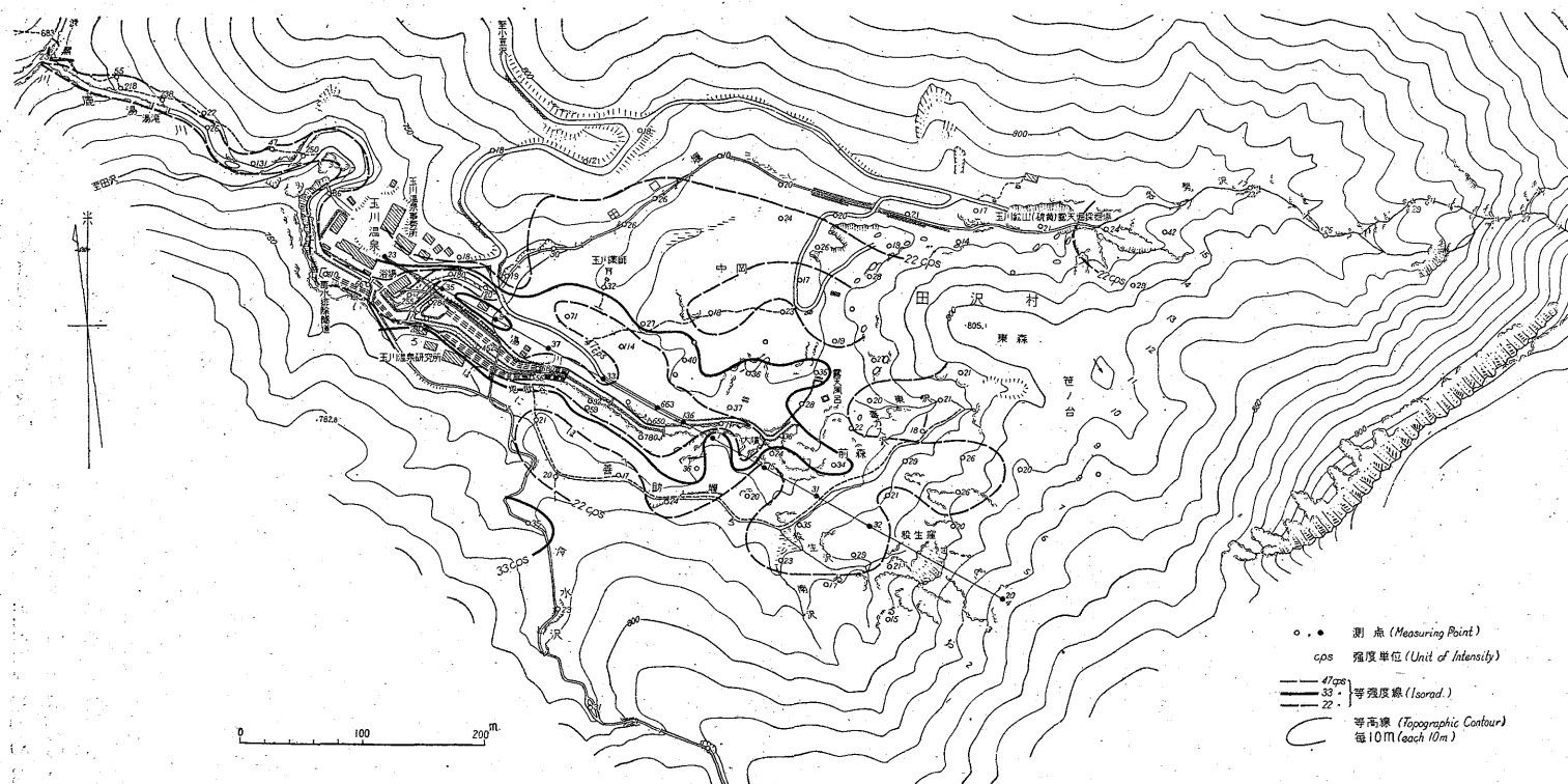
第7図 放射能強度分布図 Isorad Map at Tamagawa Hot Spring
