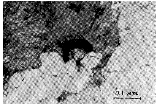
図版2a エナ石とトリウムハロ (C7) 鉱物のまわりに黄色ハロがありさらに Th ハロがかこむ
