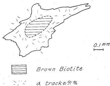
第 4 図 周辺部が緑色の黒雲母中の放射能分布
