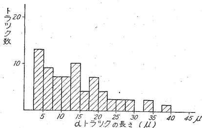
第5図 C7中のエナ石によるαトラツクの長さの割合
