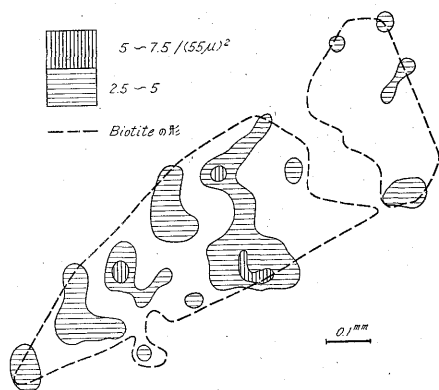
第 3 図 C5 花崗岩中の黒雲母の放射能分布図 (28 日露出)
