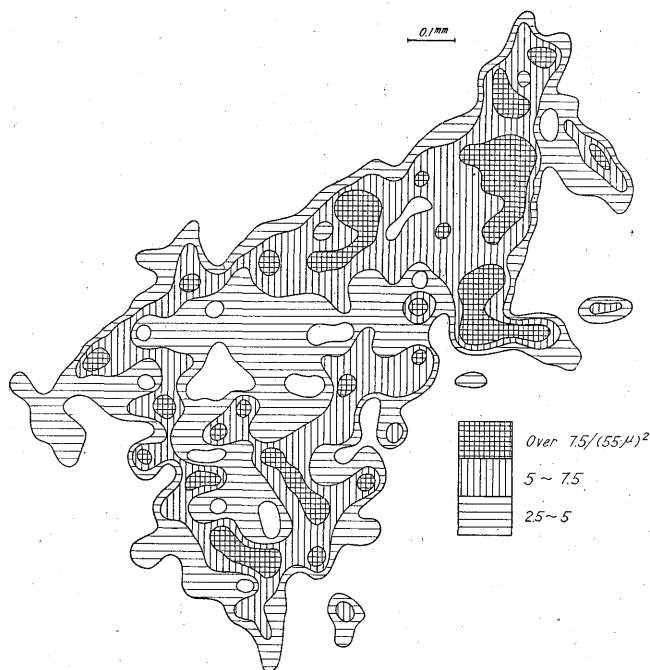
第 1 図 C5 花崗岩中の黒雲母の放射能分布図 (28 日露出)
