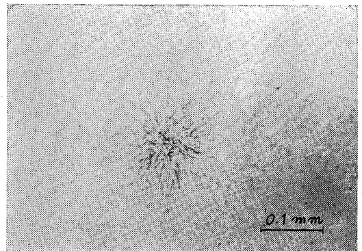
図版2b aの鉱物の4日21時間露出
