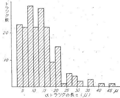
第6図 C7中のエナ石によるαトラツクの長さの割合
