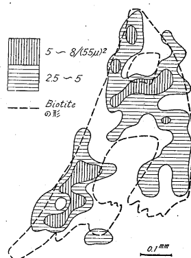
第 2 図 C5 花崗岩中の黒雲母の放射能分布図 (28 日露出)
