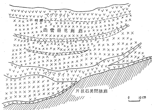
第10図 片状石英閃緑岩と両雲母花崗岩、ペグマタイト状態(玉川村蟹沢の東方道路切制)
