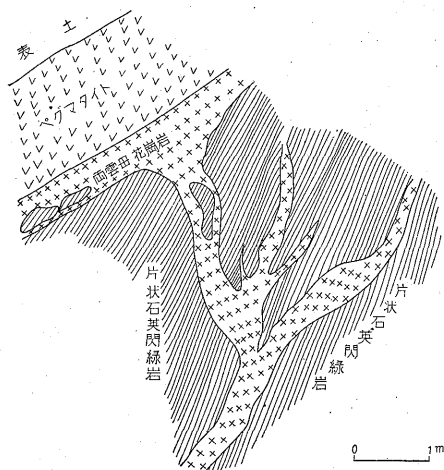
第8図 片状石英閃緑岩に貫入した両雲母花崗岩とペグマタイトとの状態(玉川村橋作東方道路切制)
