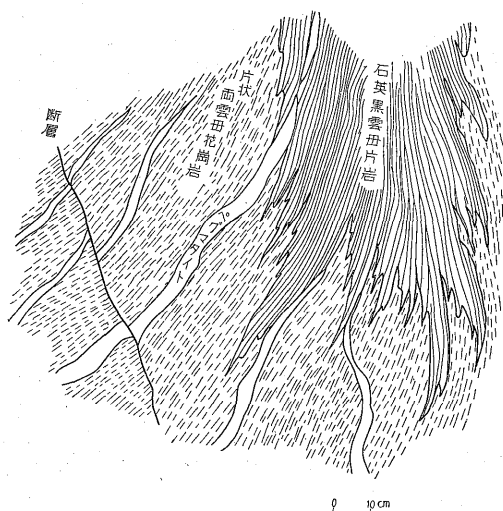
第9図 石英黒雲母片岩と片状両雲母花崗岩との接触状況(田村町坂下南方の道路切制)
