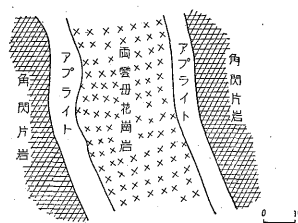
第11図 角閃片岩に貫入した両雲母花崗岩とアプライトの状態(蝦夷ガ嶽西方道路切制)
