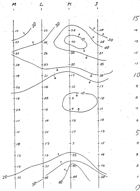
第3図 鹿の子地区比抵抗分布図 (2 極法 a=20 m)
