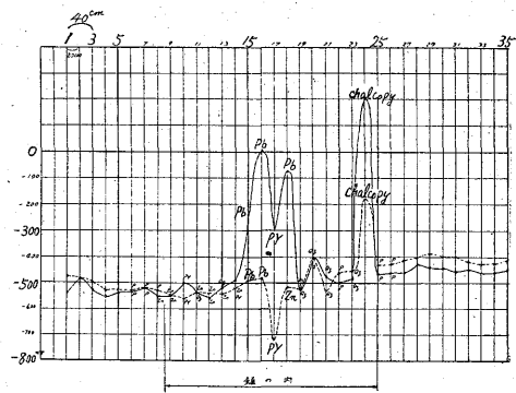
第 18 図 天神立入地質および電位断面図
