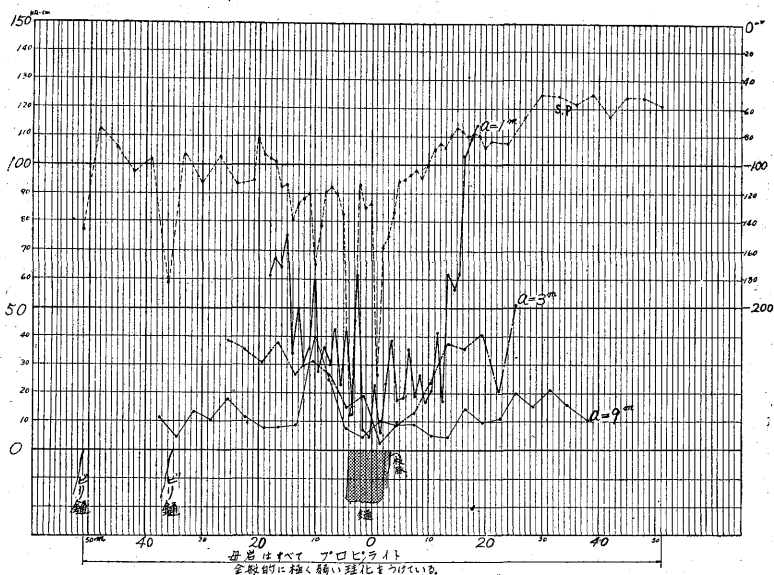
第14図 通洞鹿の子本鍾向立入坑道における坑壁測定結果
