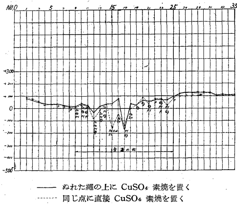
第21図 坑内実験(2) 硫酸銅電極の接触電位測定
