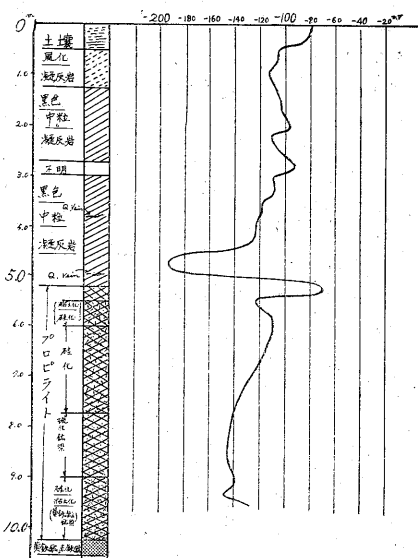
第10図 L-7 Bore Hole 内 SP-Logging
