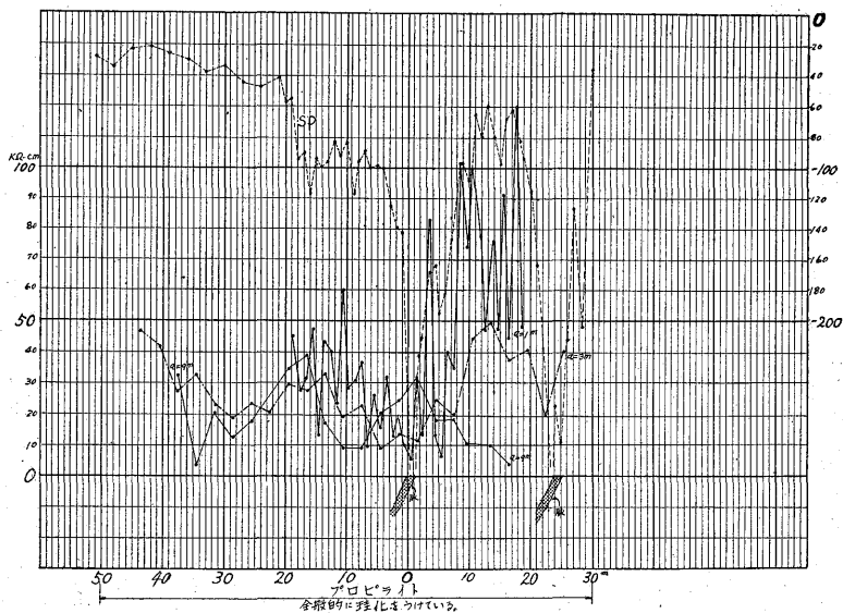
第15図 上1坑鹿の子本鍾向立入坑道における坑壁測定結果
