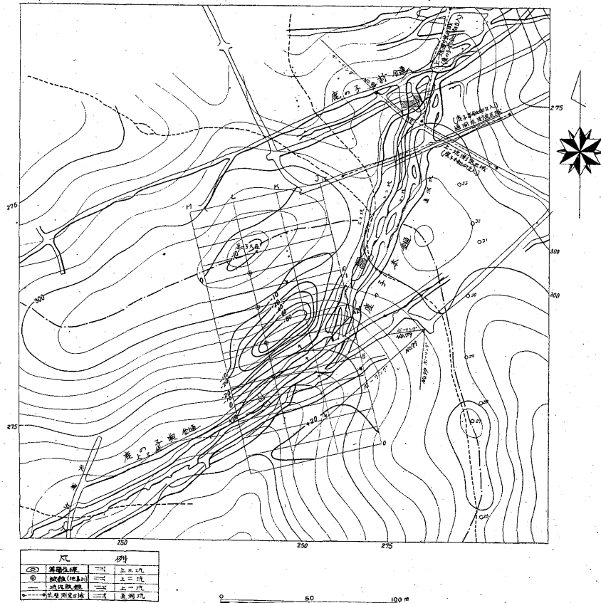
第1図 細倉鉾山麓の子鉾床上部等電位線図
