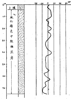
第12図 L-11 Bore Hole 内 SP-Logging
