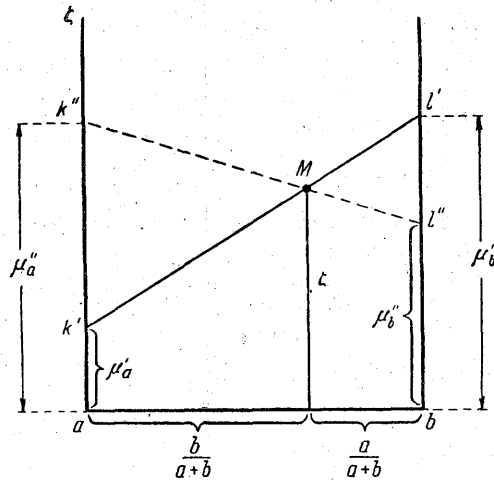
第54図 2成分結合物 M の化学ポテンシャルの相関関係を示す
