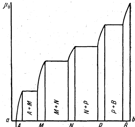
第60図 第59図と同様であるが、可変組成の鉱物をもっている
