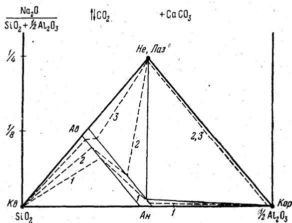
第63図 方解石過剰の場合の \text{SiO}_2-\frac{1}{2}\text{Al}_2\text{O}_3-\text{Na}_2\text{O} 系(東部シベリアの古生代鉱物相)におけるナトリウムの等ポテンシャル線 Ab: 曹長石, An: 灰長石, Kb: 石英, Kor: 鋼玉, Laz: 青金石, Ne: 霞石
