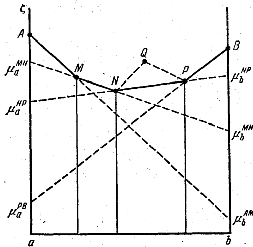
第55図 一定成分 A, M, N, P, B 鉱物を含む2成分系内における成分の化学ポテンシャル \mu_b と組成との結び付きを示す
