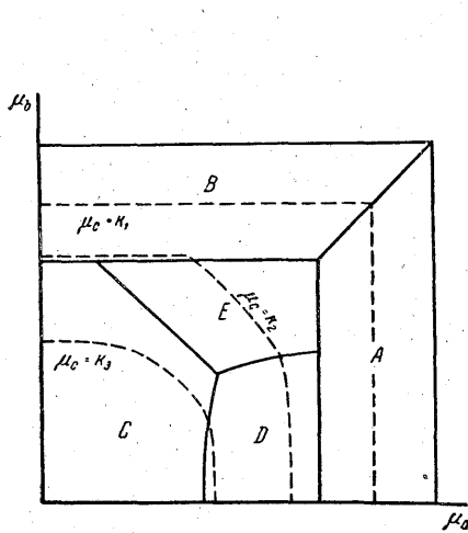
第70図 \frac{a}{c} - \frac{b}{c} の組成-共生関係の濃度図表
