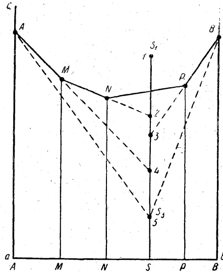
第 64 図 S 鉱物の a, b 不活性成分の化学的ポテンシャルの逐次低下, 完全移動成分 c — 鉱物 S にのみ含まれている — の化学的ポテンシャルの上昇とは、 a-b 系における共生関係の逐次変化を誘導する。
