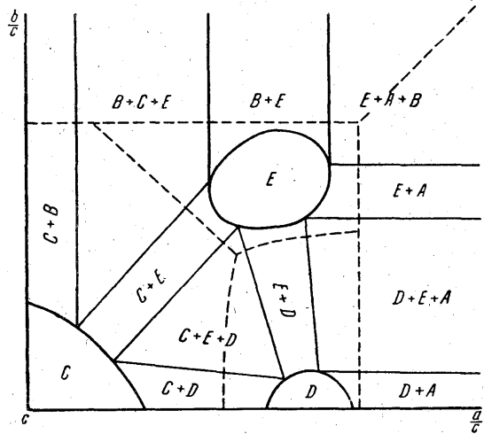
第71図 第70図の組成-共生関係図表に対応する化学的ポテンシャル面 \mu_a - \mu_b の投影図
