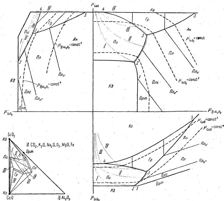
第72図 Turin 銅鉄山のスカン帯に対する \text{H}_2\text{O} , \text{CO}_2 , \text{K}_2\text{O} , \text{Na}_2\text{O} , \text{O}_2 , \text{MgO} , \text{Fe} 完全移動下における \text{CaO}-1/2\text{Al}_2\text{O}_3-\text{SiO}_2 系の組成-共生関係図とそれに対応する化学的ポテンシャル面 ( \mu\text{Al}_2\text{O}_3-\mu\text{CaO}-\mu\text{SiO}_2 ) の3成分投影によって与えられる
