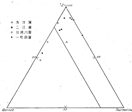
第 4 図 e 霧北層群のジルコン—電気石—柘榴石比
