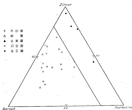
第 4 図 b 矢上層群のジルコン—電気石—柘榴石比
