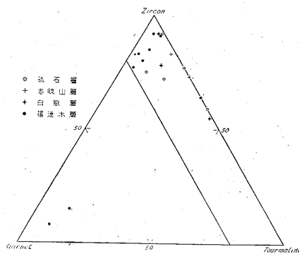
第 4 図 d 下島層群のジルコン—電気石—柘榴石比
