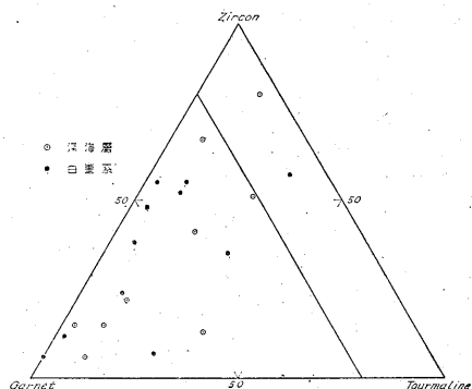
第 4 図 c 白雲系赤崎層群のジルコン—電気石—柘榴石比
