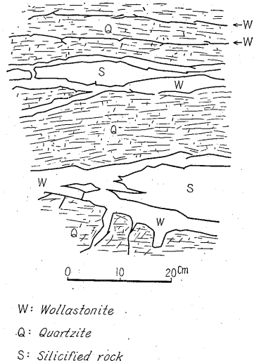
第2図 珪灰石の産状
