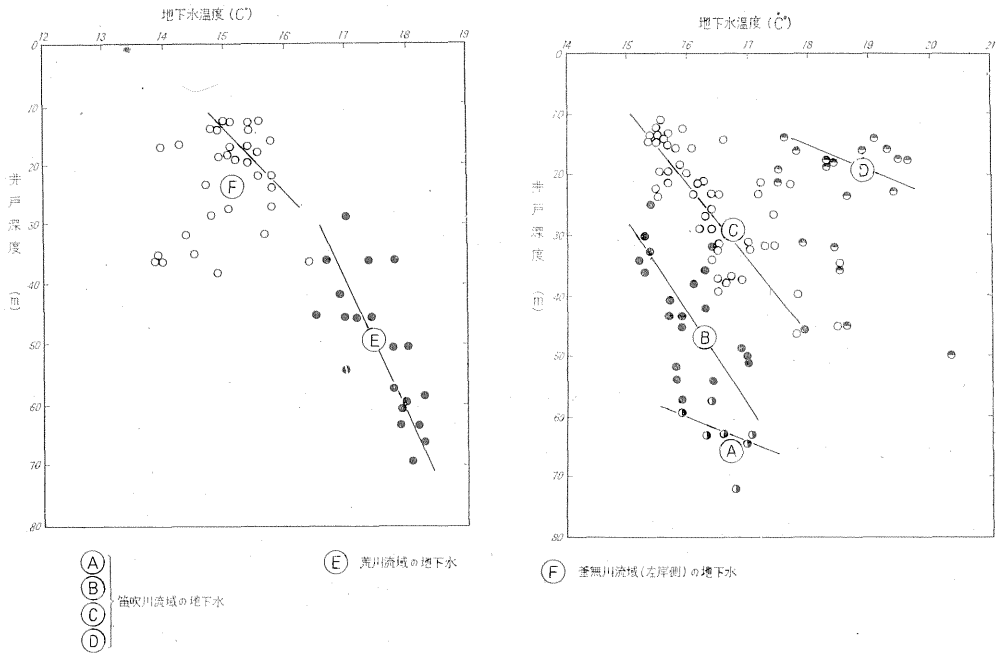
第 12 図 深度別に見た笛吹川および釜無川流域における地下水温度 (第 7 図参照)
