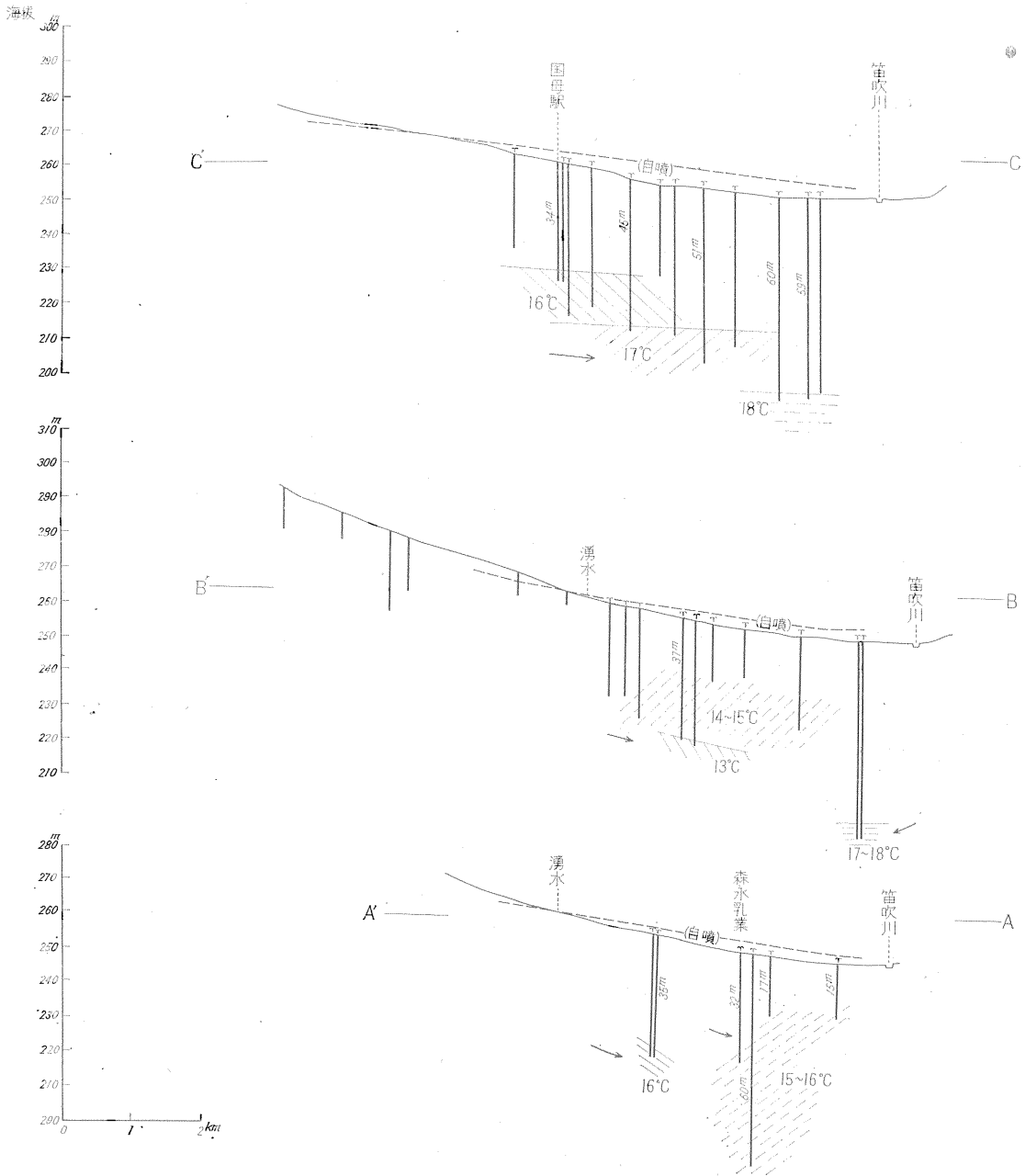
第 11 図 釜無川左岸流域の地下水温度地下断面図 (測線は第 10 図参照)
