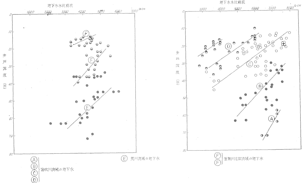
第 8 図 深度別に見た荒吹川および釜無川流域の被圧地下水水比抵抗
