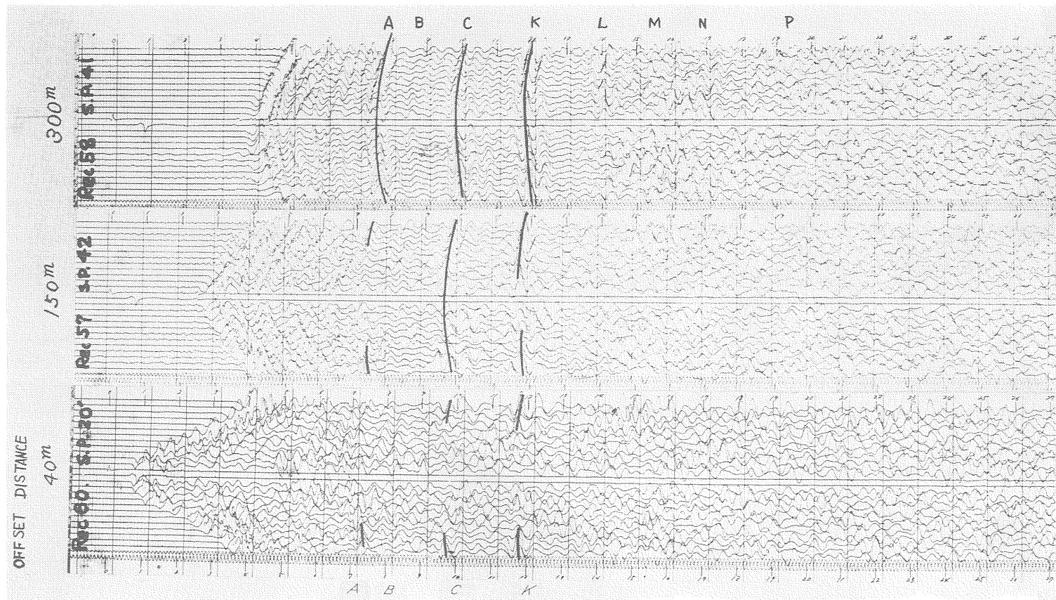
図 版 2 OFF-SET 距離を変えた場合の反射記録の変化
