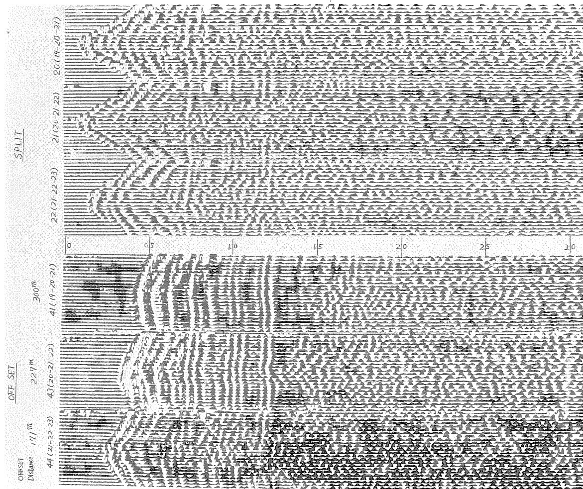
図 版 3 連続断面法における同一展開に対する SPLIT 爆破と OFF-SET 爆破との比較
