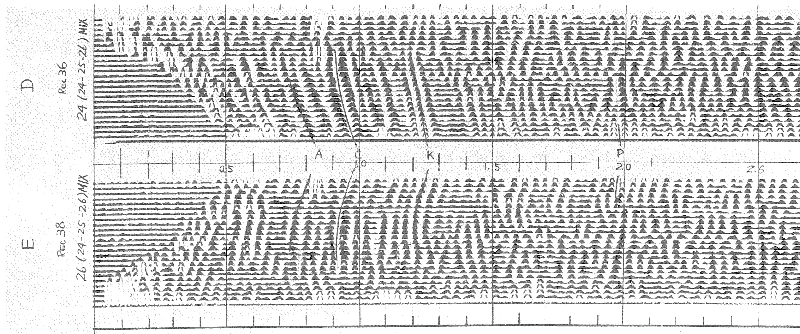
図 版 1 この地試の特有な進行性妨害波の例
