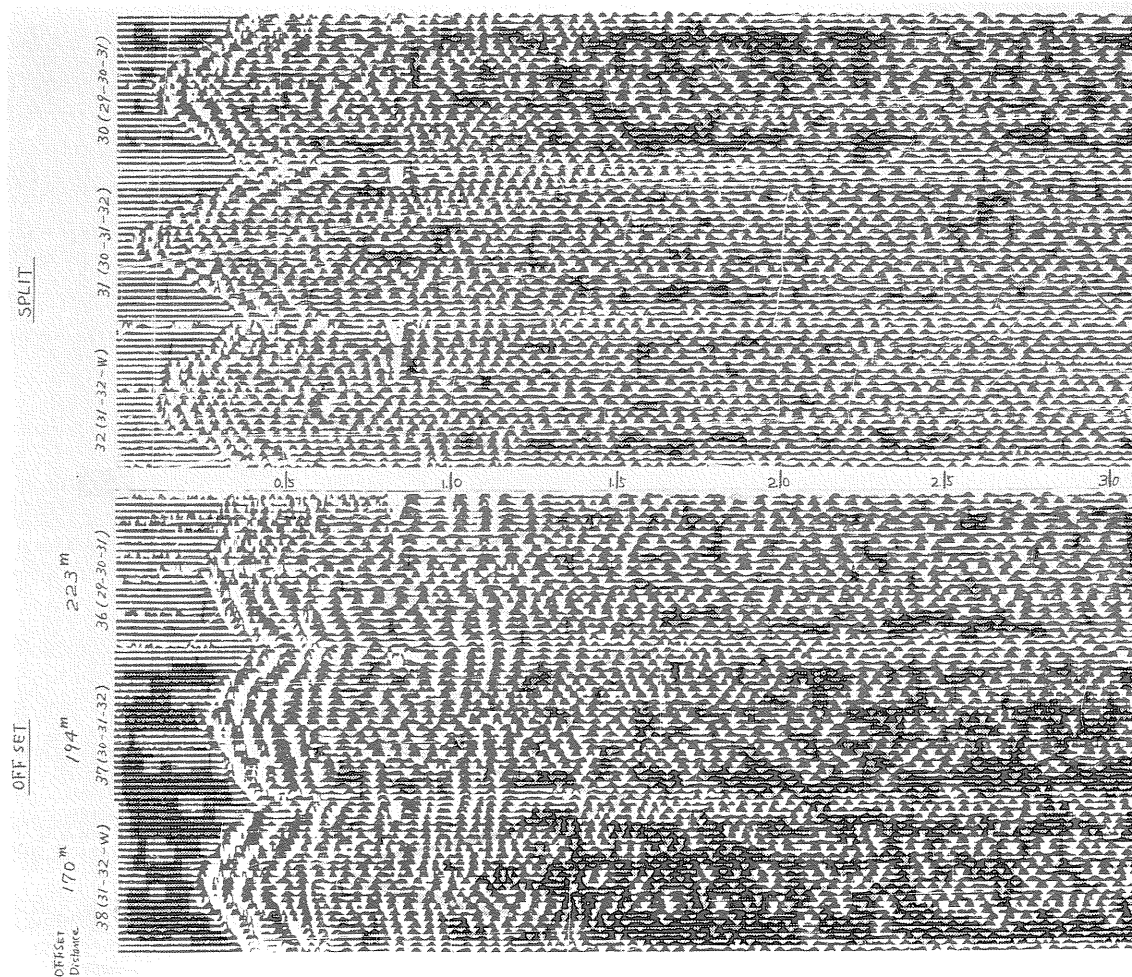
図版 4 連続断面法における同一展開に対する SPLIT 震破と OFF-SET 震破との比較
