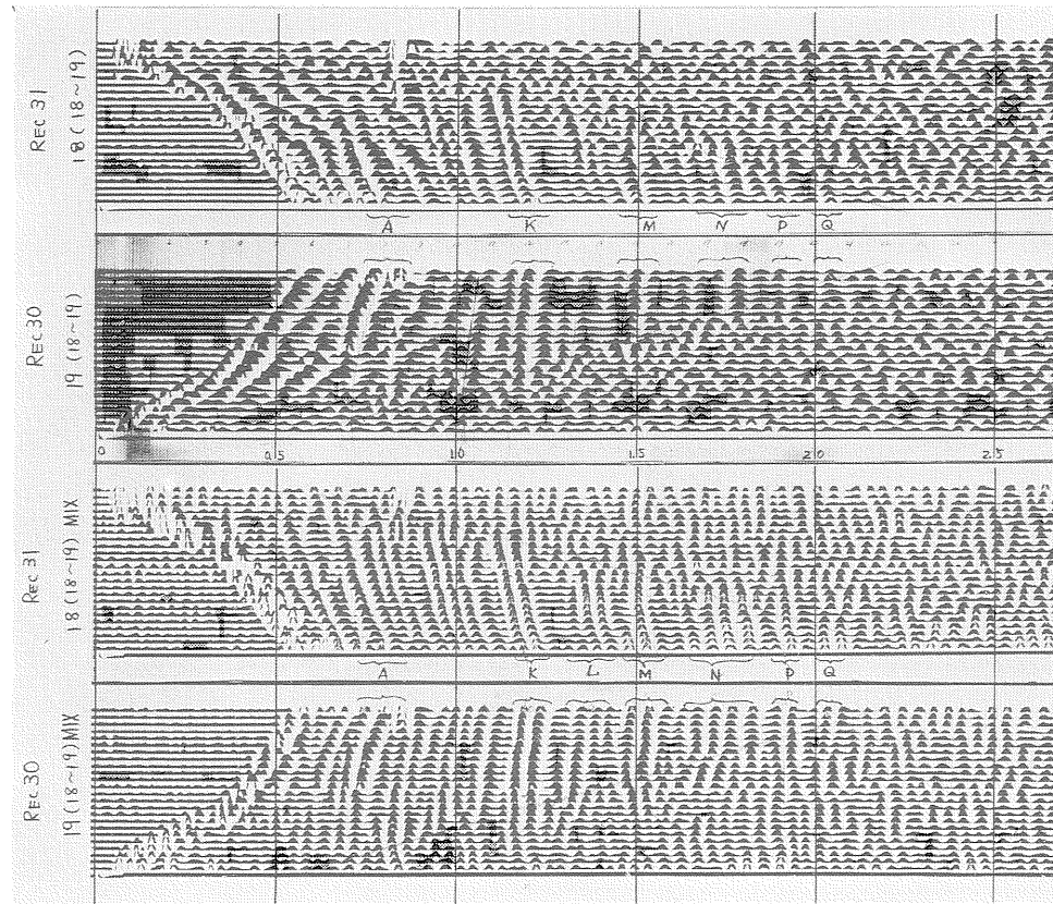
図 版 6 混合による疑似立相揃いの例, 上は混合を用いないもの, 下は混合を用いたもの
