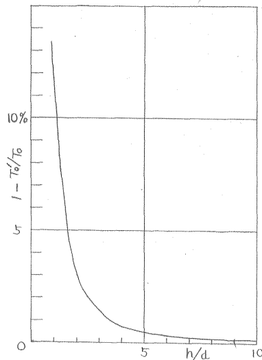
第3図 オフセット展開とスプリット展開による反射時間の变化。 T_0' , T_0 ; オフセット展開, スプリット展開における中点反射時間
