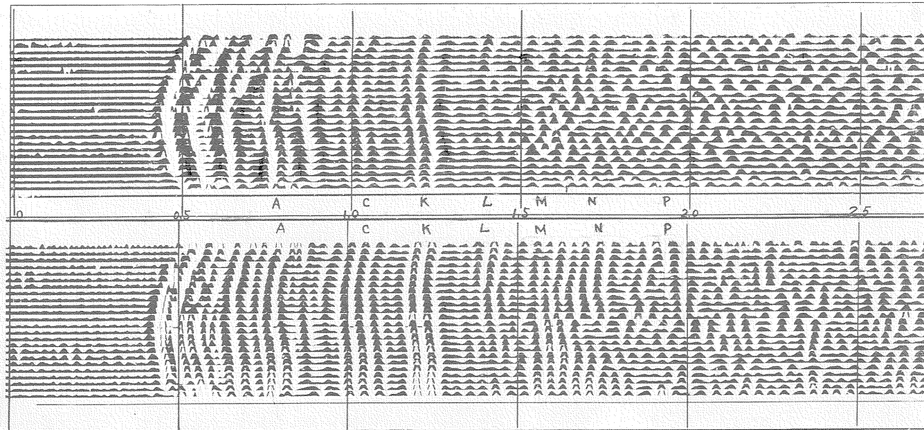
図版7 混合による反射波位相揃いの向上の例
