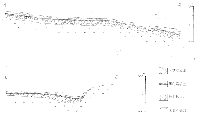
第 9 図 佐嘉鉾山第5坑断面図
