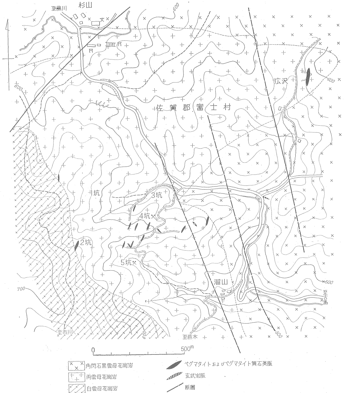
第 2 図 佐嘉鉾山付近地質図
