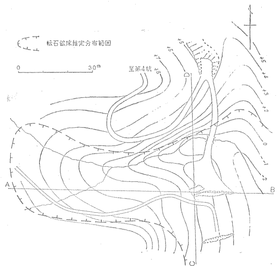
第 8 図 佐嘉鉾山第5坑平面図
