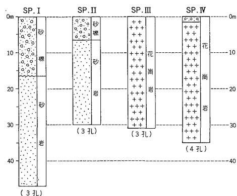
第4図 水沢周辺地震探査発破孔柱状図
