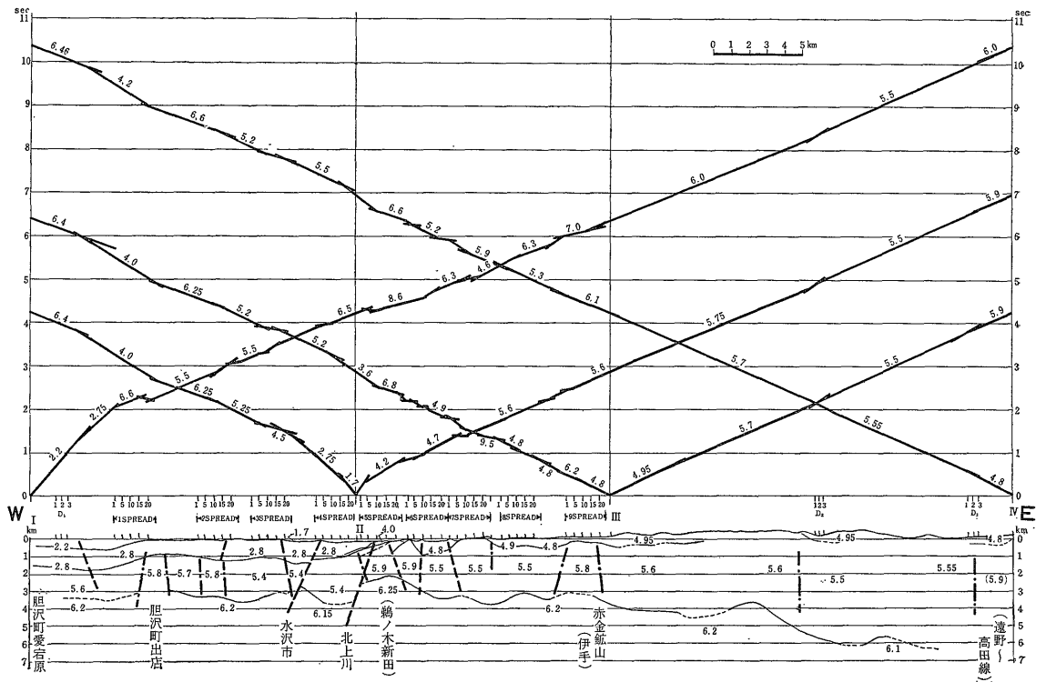
第6図b 水沢周辺地震探査走時曲線および解析構造断面図
