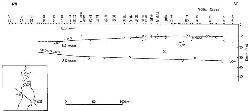
第8図 爆破地震動グループが行なった東北地方の地殻構造 (1966)
