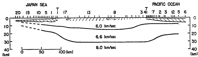
第 8 図 気仙沼沖, 土畑, 男鹿半島沖爆破により求められた東北日本の地殻構造 (Hashizume et al., 1968).
