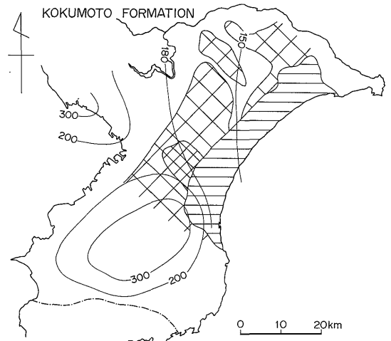
第8図 国本層の等層厚線図（単位はm）
