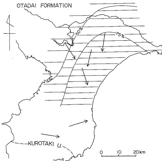
第5図 大田代層堆積時の古環境
