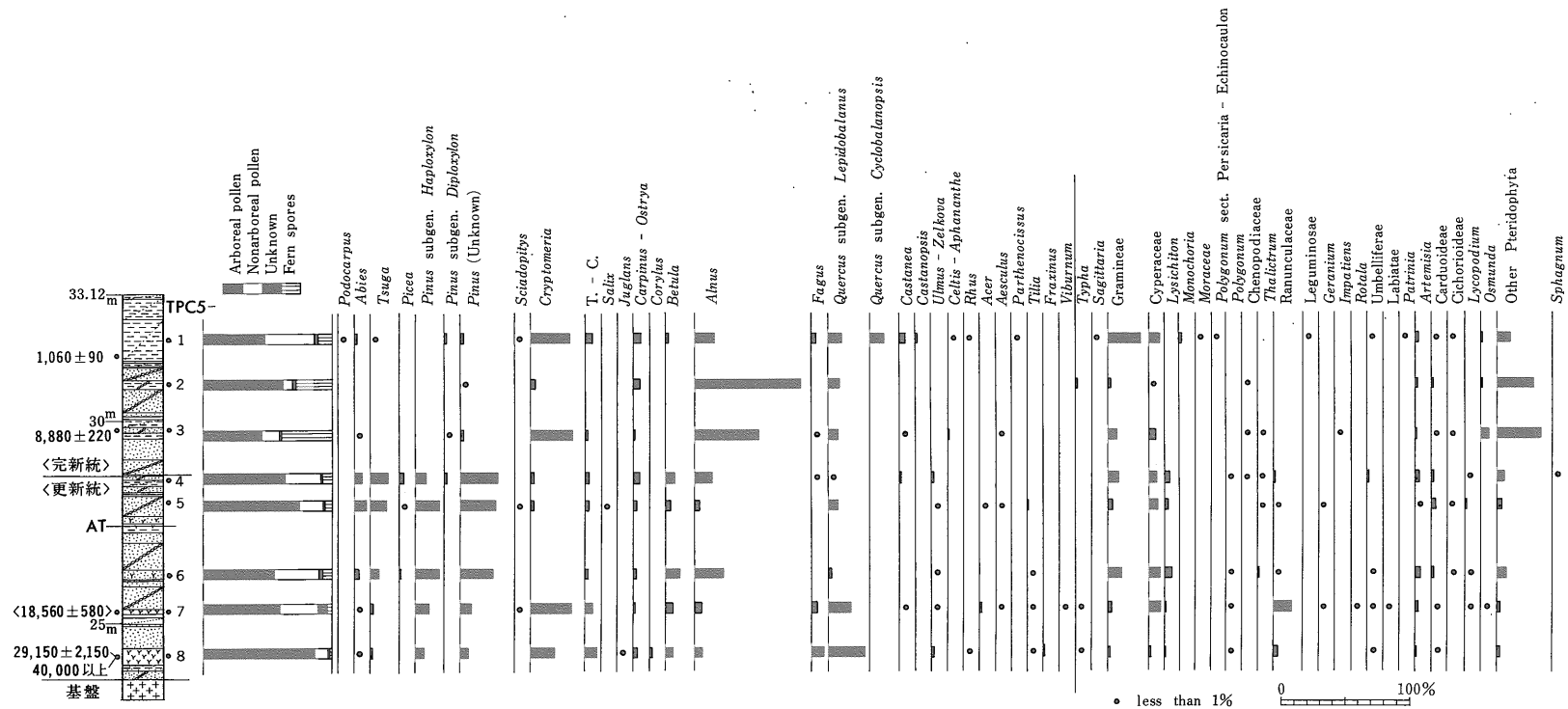
第 17 図 C-5 ボーリング試料の花粉ダイアグラム
