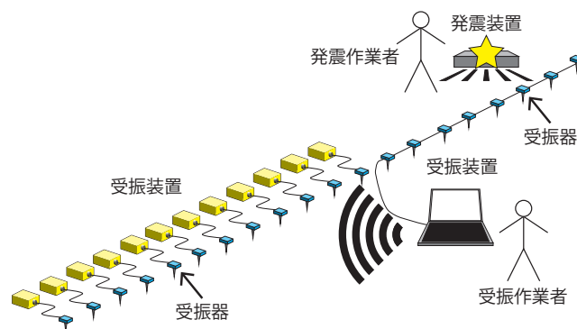
第1図 反射法地震探査の概念図。作業は発震に関わるものと受振に関わるものに大別される。後述するように発震装置・受振装置には様々なものがある。
